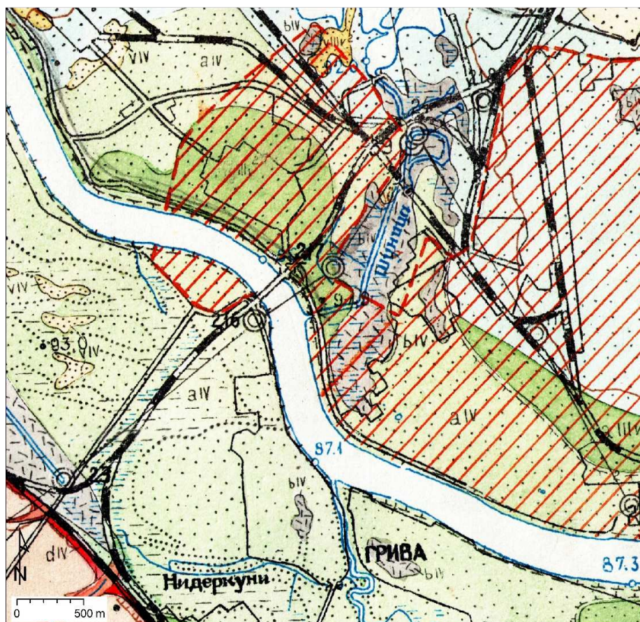
7. attēls. Pūķu teritorijas un piegulošās teritorijas kvartāra nogulumu karte (datu avots: Juškevičs et al., 1978)
