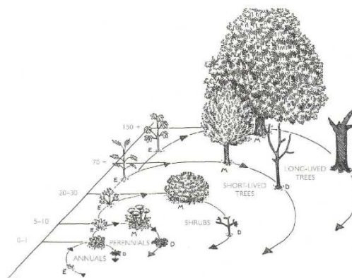
73. attēls. Veģetācijas attīstība pa gadiem
