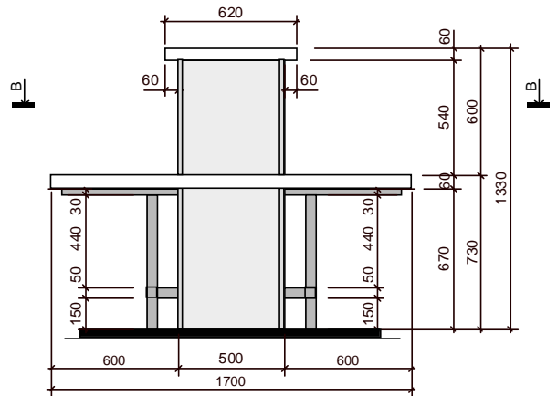
Griezums A-A
