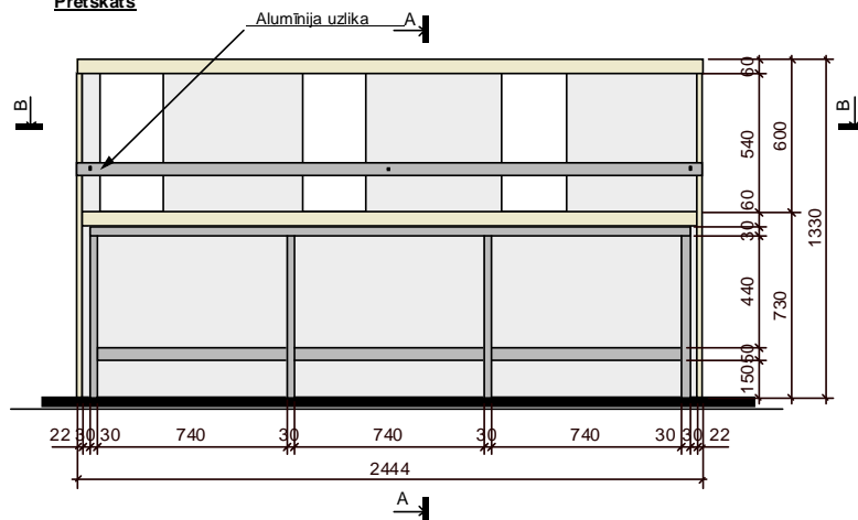
Pretskats
