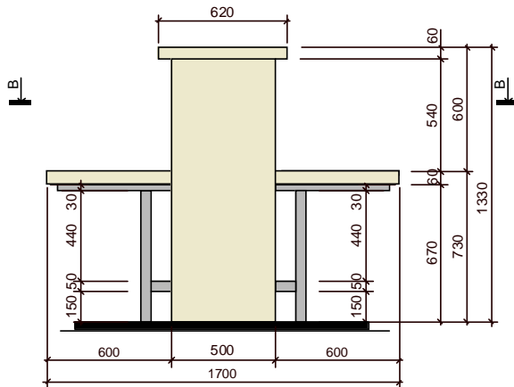
Sānskats
