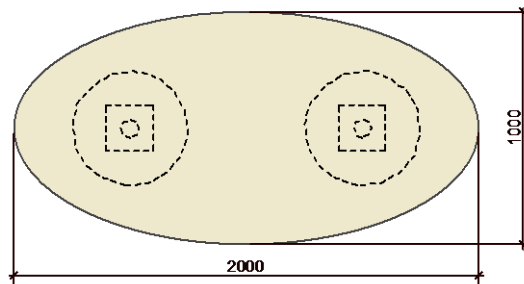
Pretskats
