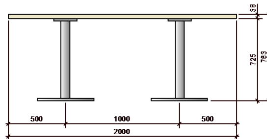
Pretskats
