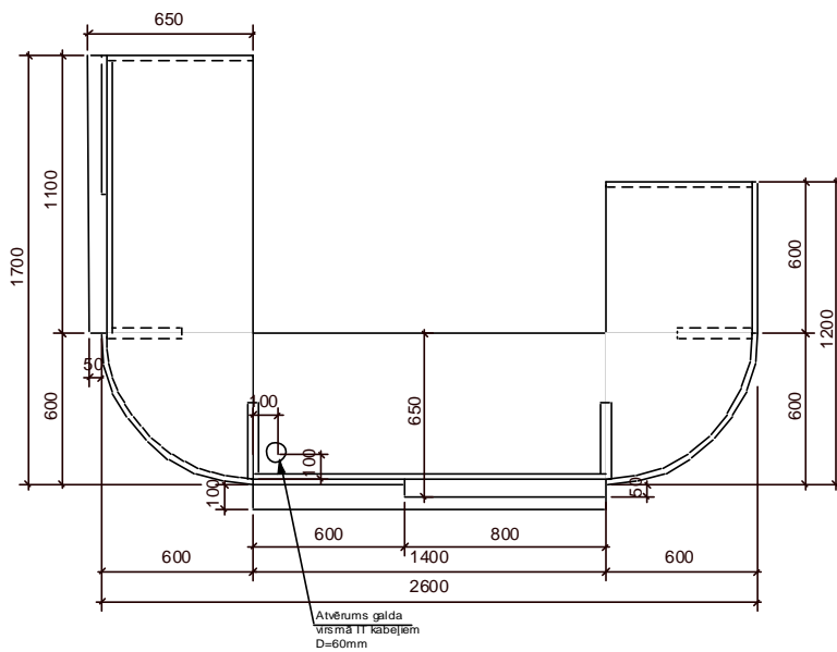
Virsskats
