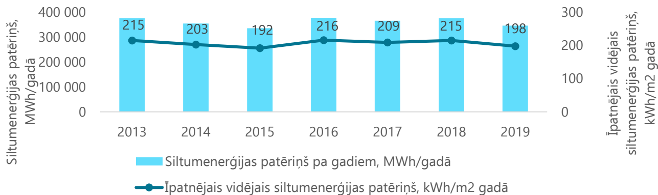
ATTĒLS 102. Kopējais siltumenerģijas patēriņš ēkās Daugavpilī un īpatnējais vidējais patēriņš gadā (Datu avots: PAS DSilt)
