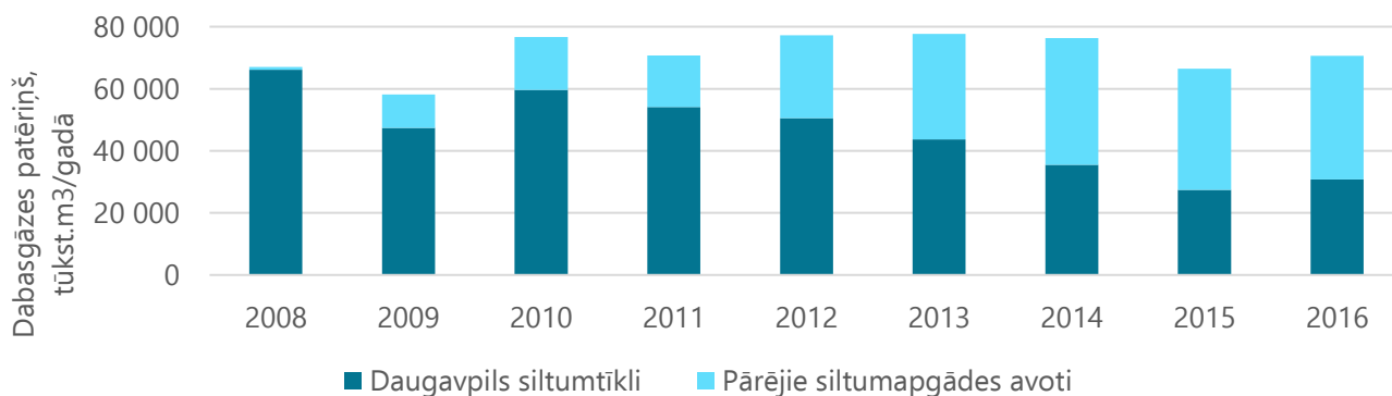
ATTĒLS 100. Dabasgāzes patēriņš siltumapgādes vajadzībām Daugavpilī (Datu avots: AS "Gasol")
