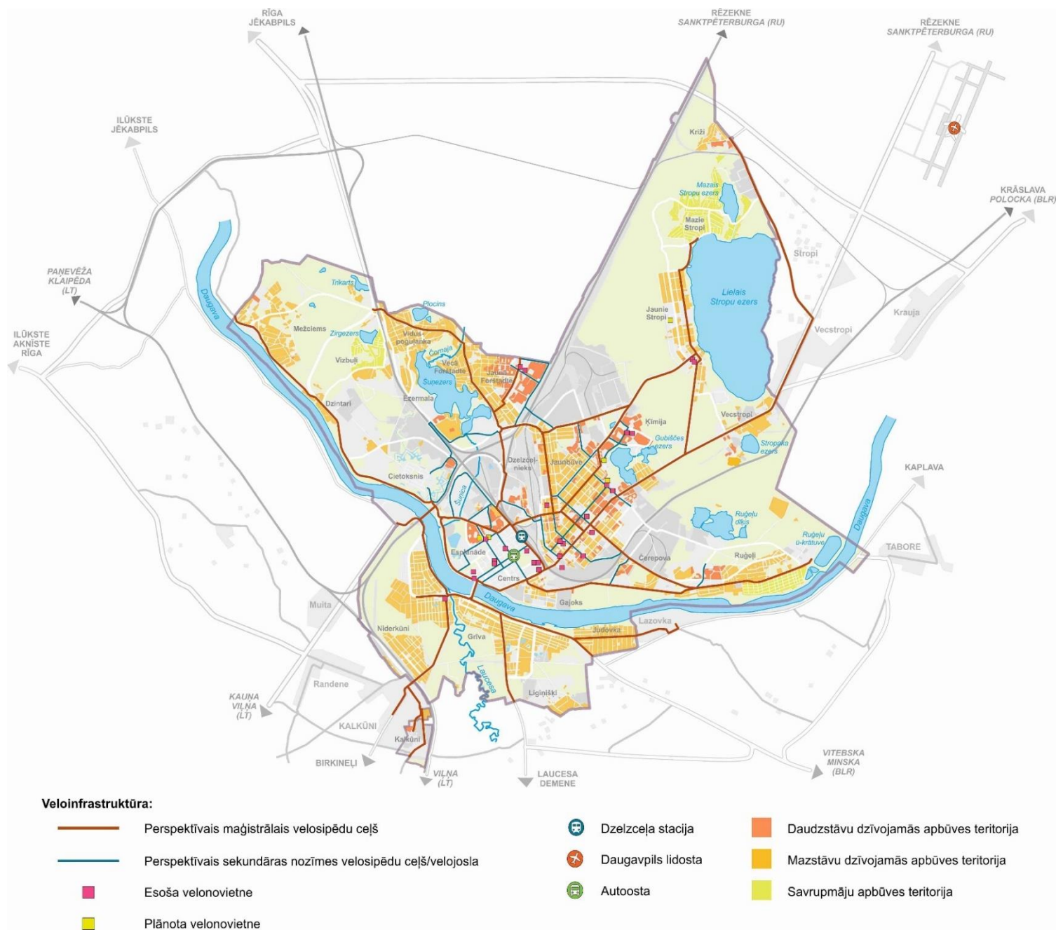
ATTĒLS 117. Velosatiksmes infrastruktūras attīstības plāns Daugavpilī (Avots: Daugavpils pilsētas teritorijas plānojums)
