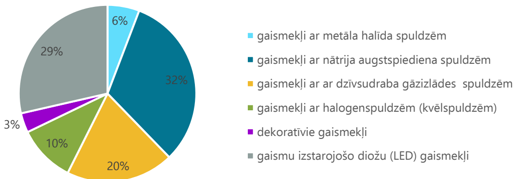
ATTĒLS 106. Gaismekļu sadalījums publiskajā ielu apgaismojumā (Datu avots: Daugavpils pilsētas attīstības departaments)
