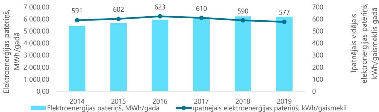
ATTĒLS 107. Kopējais elektroenerģijas patēriņš un īpatnējais patēriņš gadā (Datu avots: Daugavpils pilsētas attīstības departaments)
