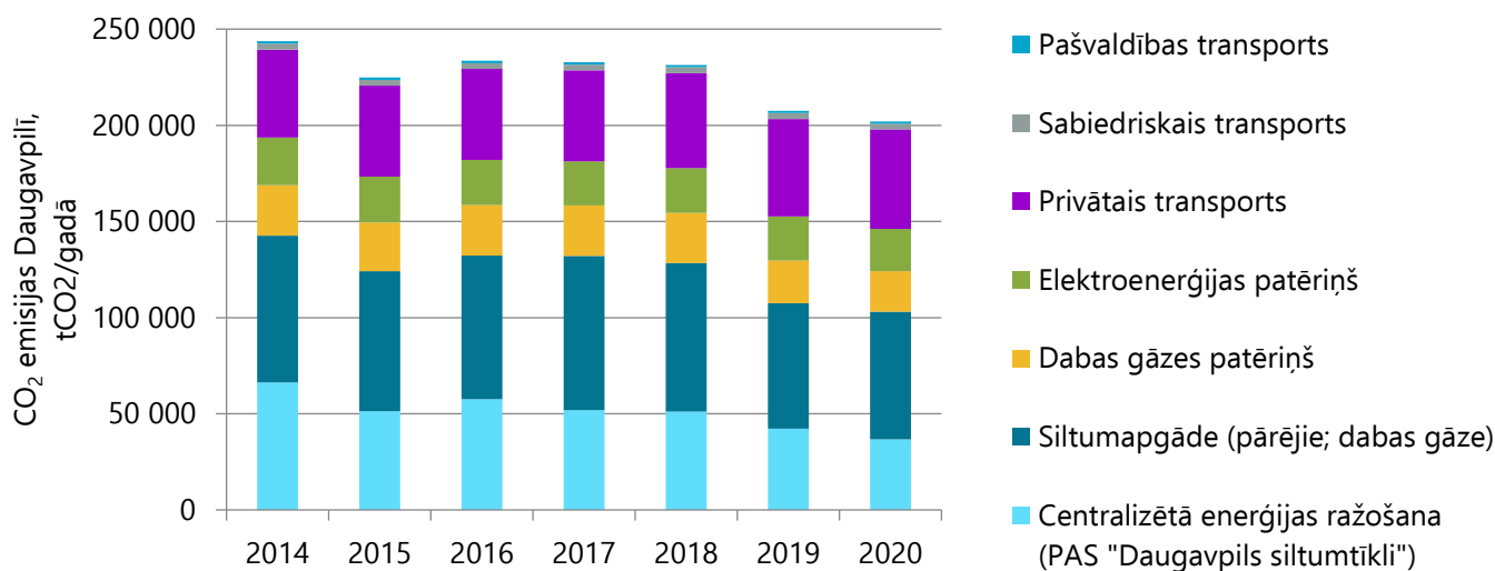
ATTĒLS 109. CO 2 emisiju apjoms Daugavpilī 2014.-2020.gadā
